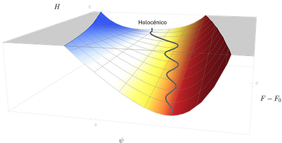
FIGURA 3. Diagrama de estabilidade do Sistema Terrestre e a sua trajetória das condições estáveis do Holocénico para um novo equilíbrio onde a temperatura média é necessariamente mais elevada. Neste diagrama, F , representa a energia livre, H , a atividade humana, \psi , a diferença de temperatura com relação a temperatura média no Holocénico.
